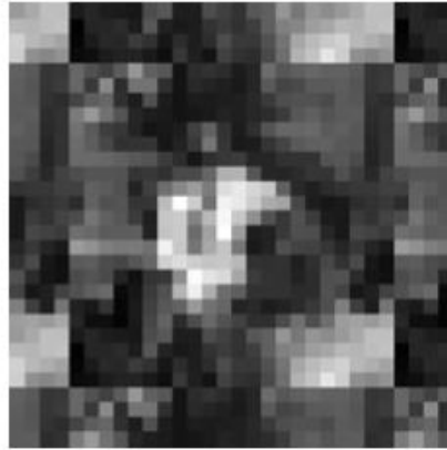
wrap
