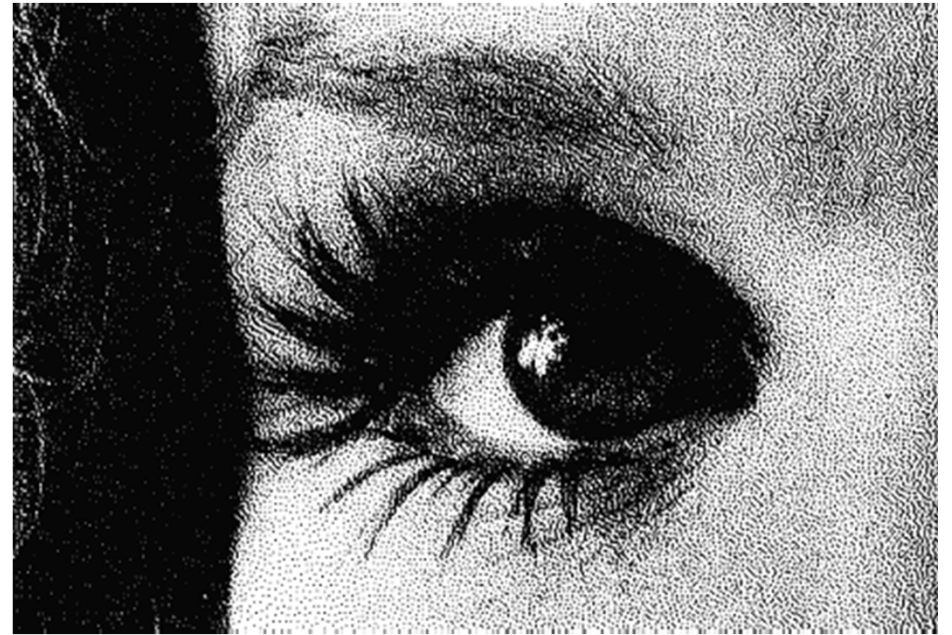
Dithering
