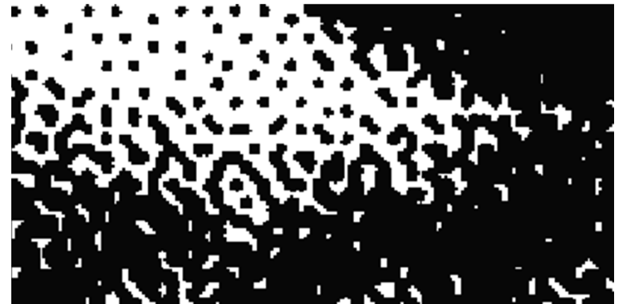
Dithering
