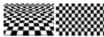
Texture Gradient
