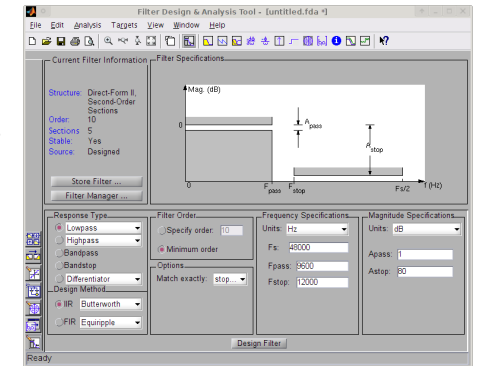
MATLAB fdatool
