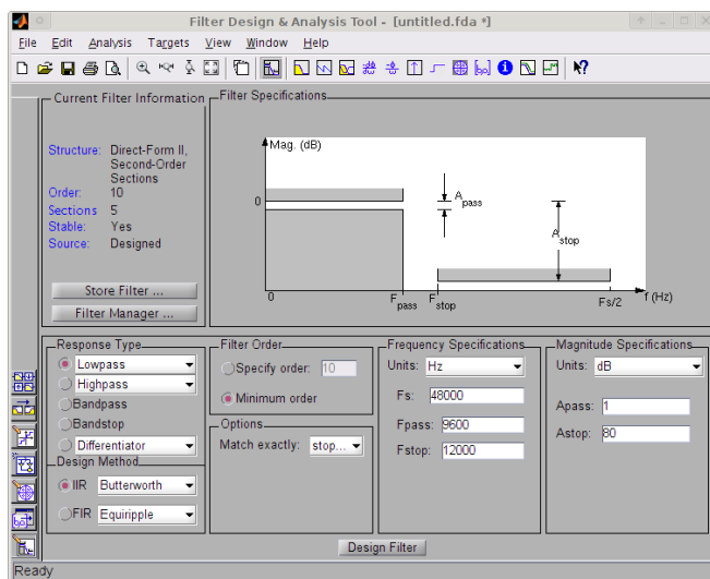
MATLAB fdatool
